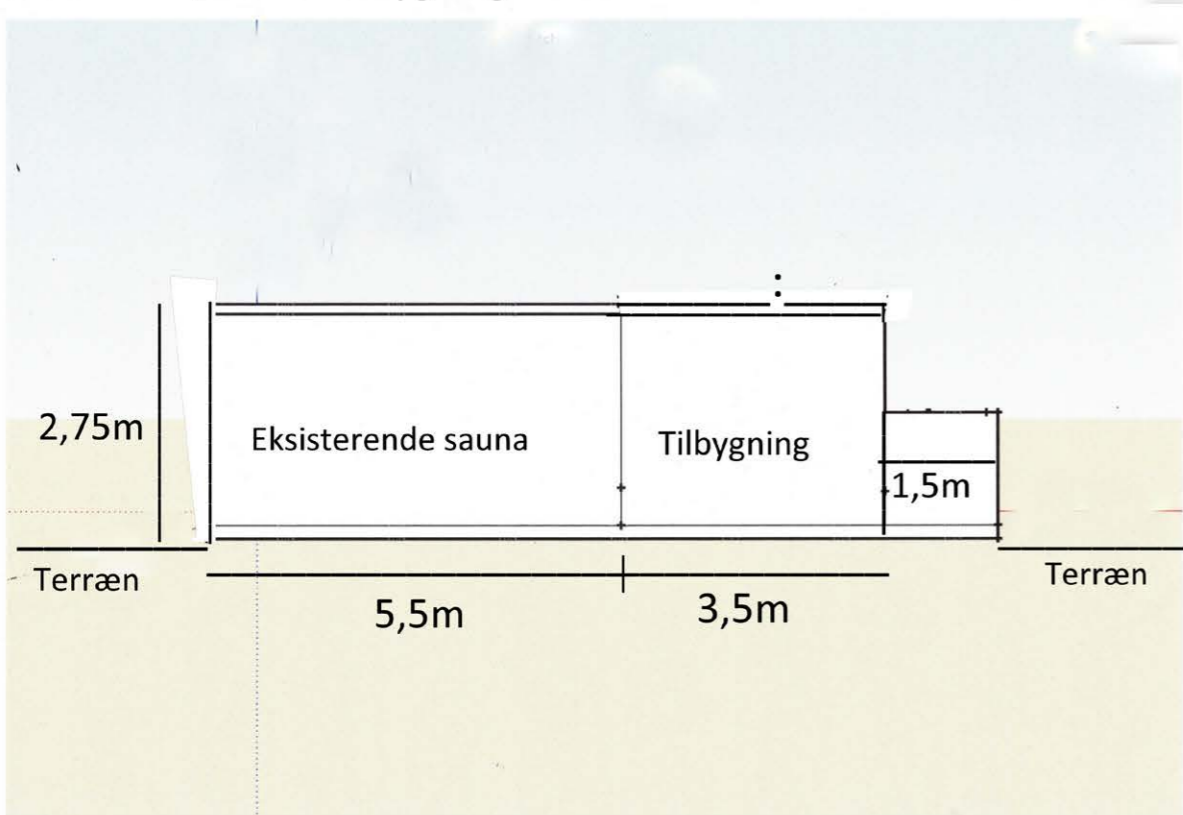
Facade mod syd efter tilbygning
