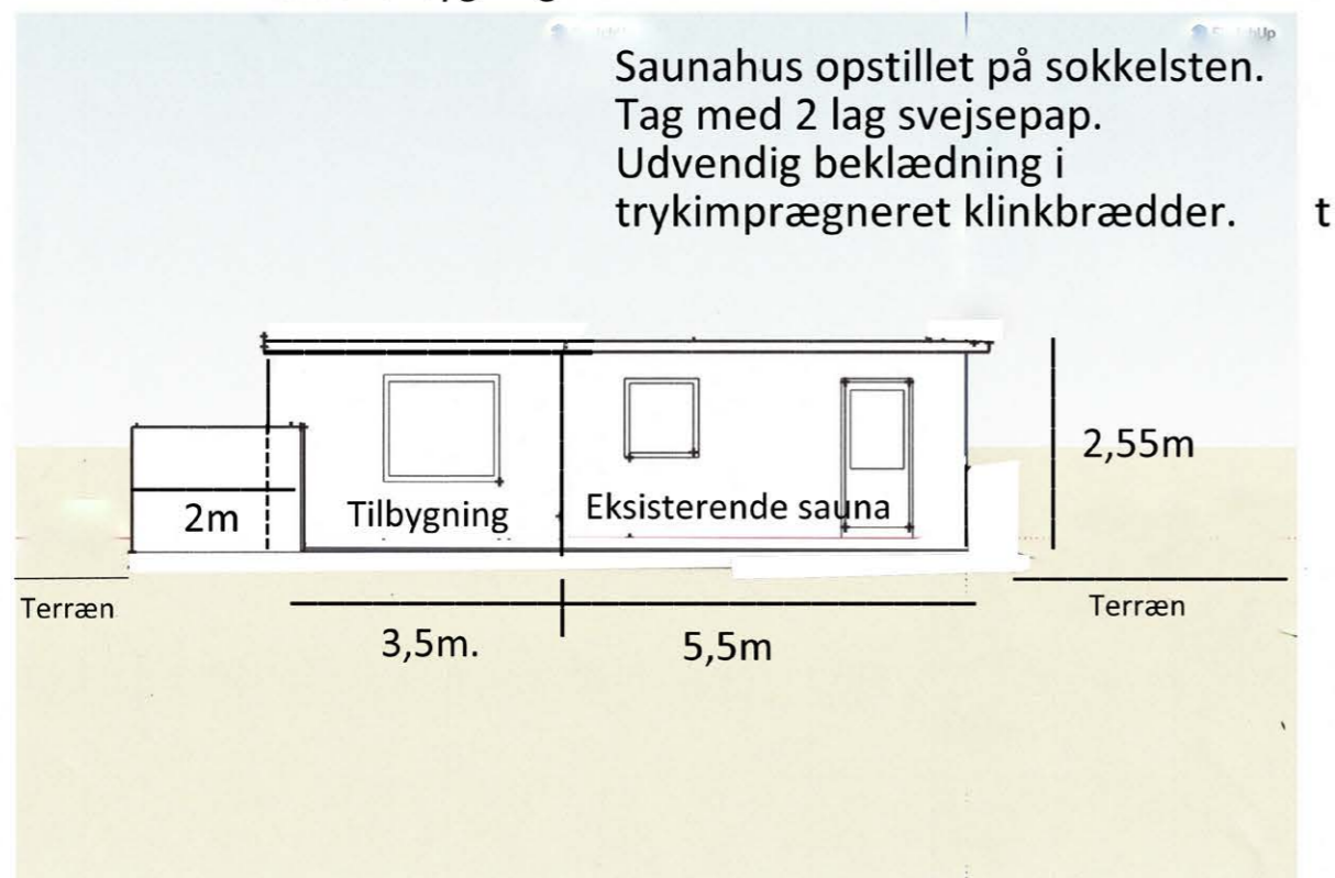
Facade mod nord efter tilbygning
